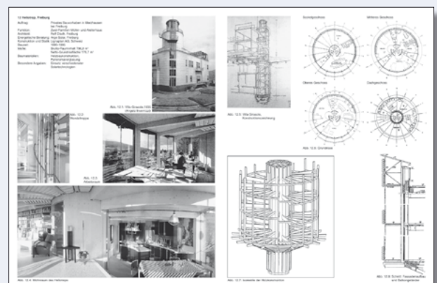
Heliotrop (Zwei-Familien-Wohn- und Atelierhaus), Freiburg (1993–95)
